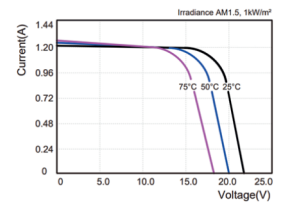
Curvas I-V del módulo PV ESF-20MF a varias temperaturas de celda I-V Curves of PV module ESF-20MF at various cell temperatures
