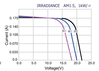
Curvas I-V del módulo PV ESF-3PC a varias temperaturas de célula I-V Curves of PV module ESF-3PC at various cell temperatures
